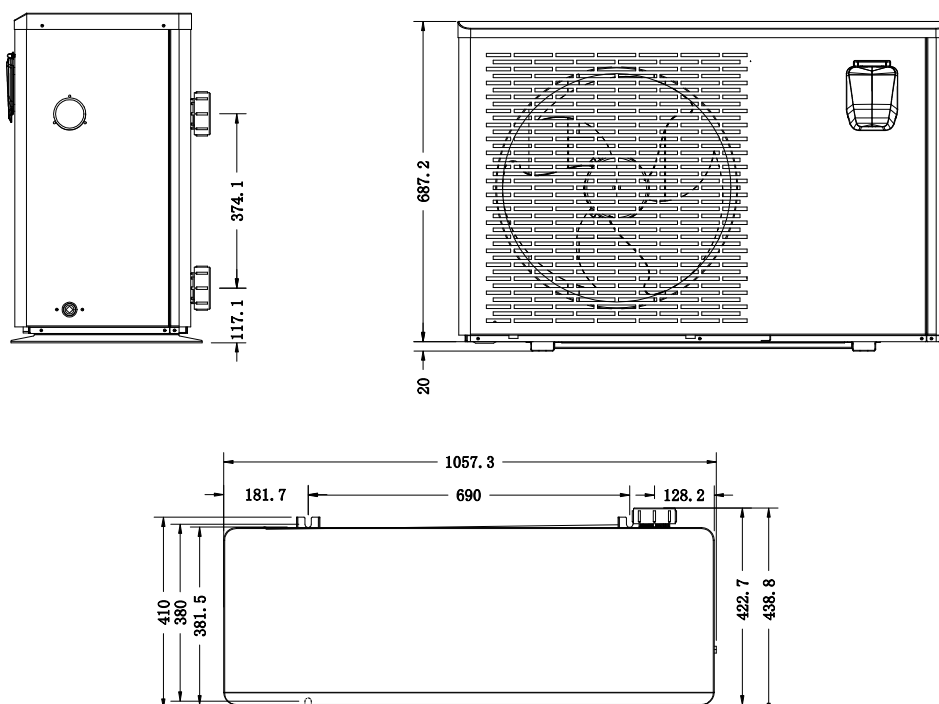
Värmepump 1402, 1403 och 1404
