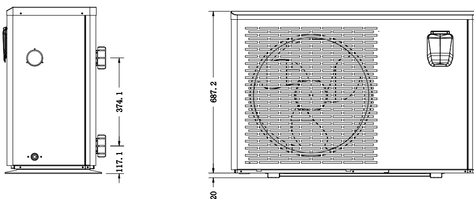
Warmtepomp 1402,1403 en 1404
